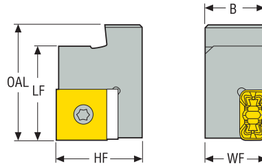
CT-PLANR/L
