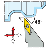
SVVBN KAPR = 72,5 °
