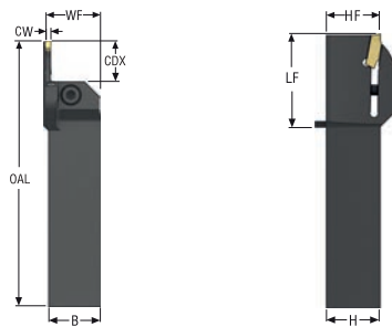
CFOR...L...JETI, CFOL...R...JETI
