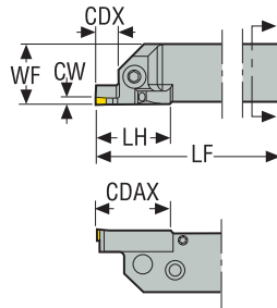
CFIR...R...JET, CFIL...L...JET
