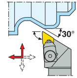
CDNNN KAPR = 62,5 °
