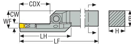
CFOR...L...JET, CFOL...R...JET
